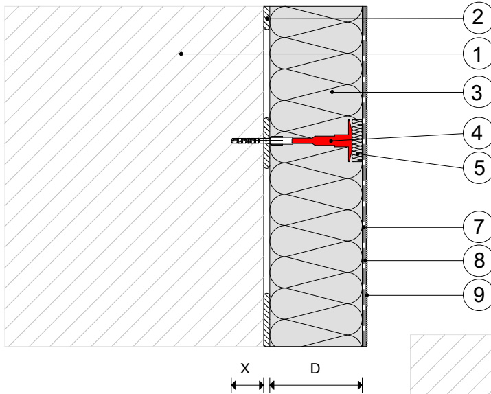
a) Baunit SchraubDübel Speed mit Rondelle
